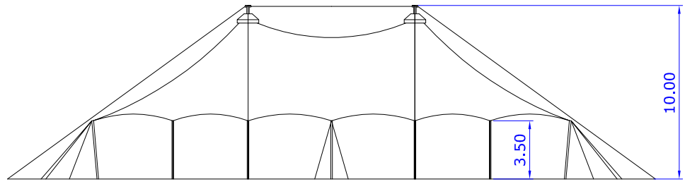
PROSPETTI
